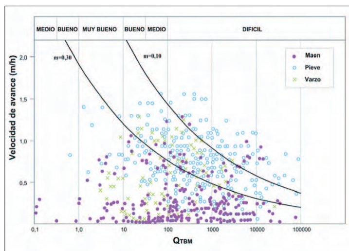
[Figura A] Velocidad de avance para tres túneles construidos con tuneladora en función de Q_{TBM} (Sapigni et al. 2002).
