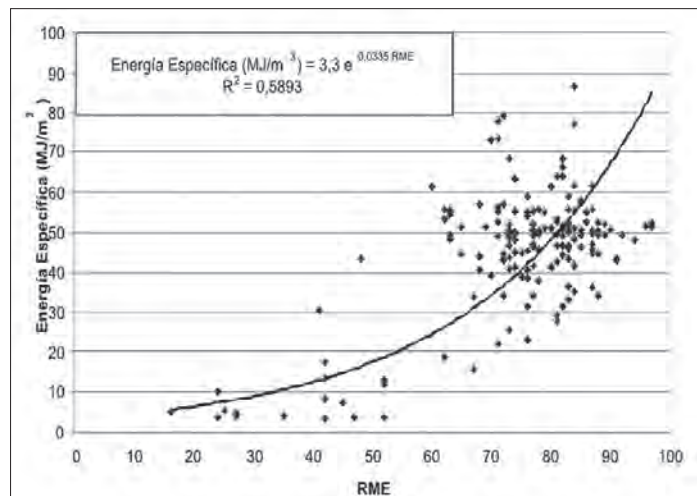
[Figura 5] Correlación entre el RME y Energía Específica.
