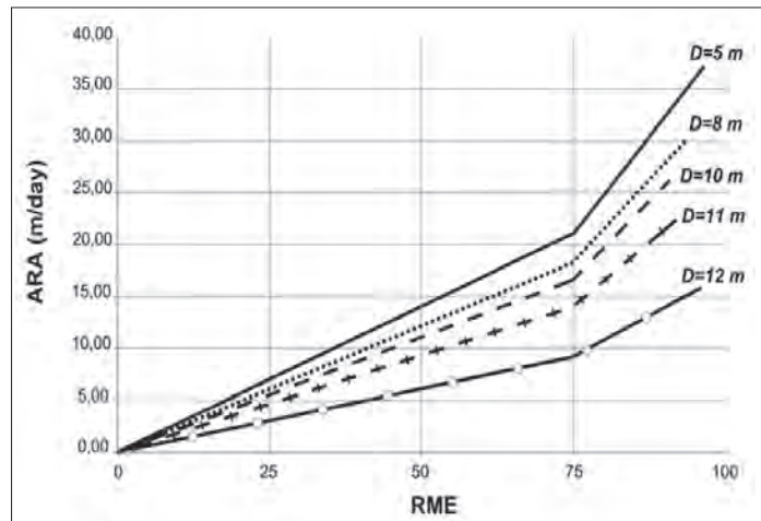
[Figura 4] Correlación entre ARA (m/día) y RME para distintos diámetros de excavación.
