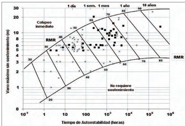
[Figura 2] Tiempo de autoestabilidad en función del RMR y de la máxima distancia sin sostenimiento.
