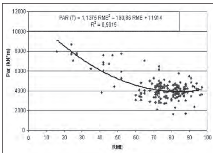
[Figura 7]- Correlación entre el RME y el par (T) aplicado en la cabeza de corte.
