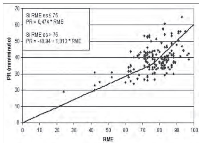
[Figura 6]- Correlación entre el RME y la Penetración Neta.
