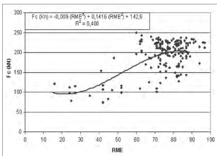
[Figura 8]- Correlación entre el RME y el empuje por cortador aplicado en la cabeza de corte.
