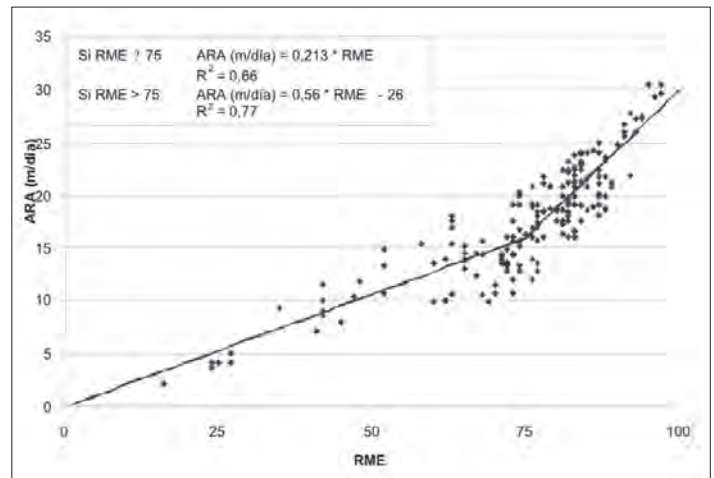
[Figura 3] Correlación entre ARA (m/día) y RME .
